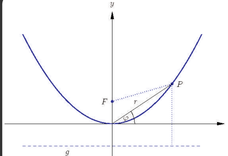
Parabola
