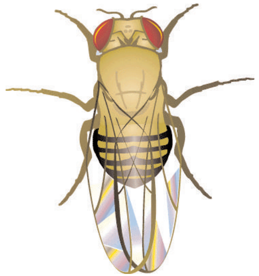
Drosophila
